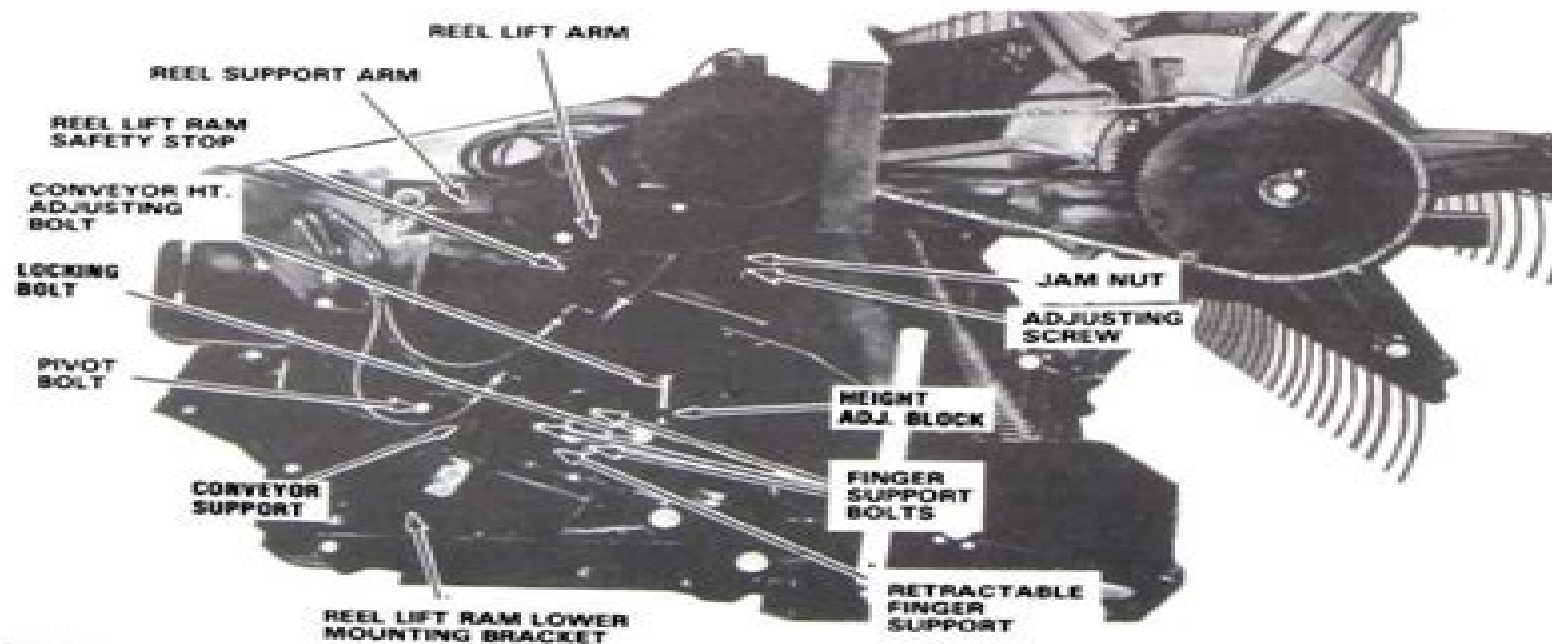
FIGURE 5 - R.H. End
